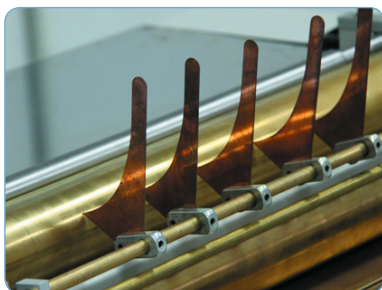
Rodillo de aplicación de cola y cubeta fabricados en aleación de cobre
