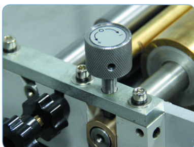
Ajuste mecánico de espesor de cola.
